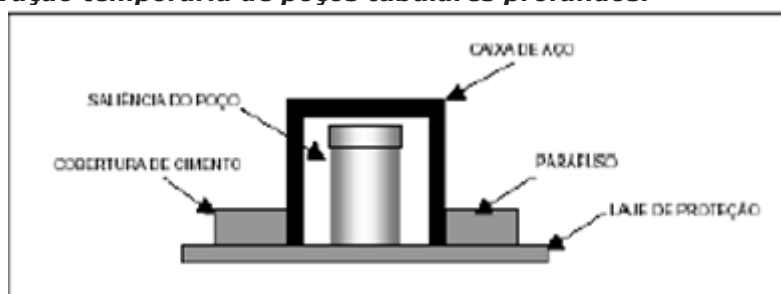
Figura 4 – Esquema de caixa de proteção externa para proteção da cabeça do poço para desativação temporária de poços tubulares profundos.
